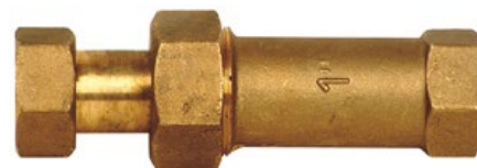
Compensador de dilatación de latón, rosca hembra-hembra 1-1/2", carrera 15mm
